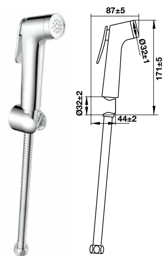
Vòi xịt vệ sinh Airsense chrome Toilet spray Airsense chrome
