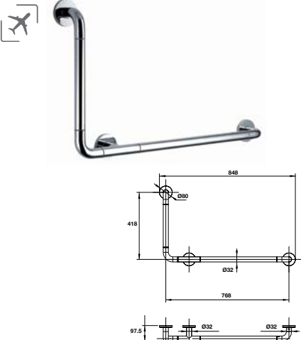
Tay vịn phòng tắm 90° 418 mm Handicapped 90° grab bar 418 mm
