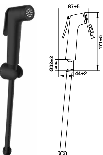
Vòi xịt vệ sinh Airsense đen Toilet spray Airsense black
