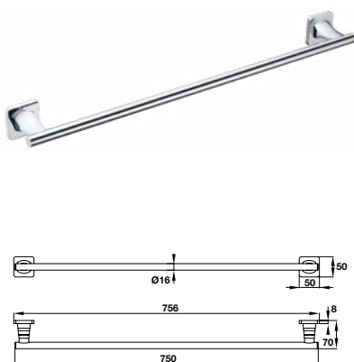
Thanh treo khăn đơn 750 mm Single towel bar 750 mm
