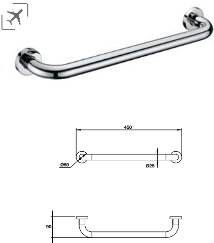
Tay vịn phòng tắm 450 mm Grab bar 450 mm
