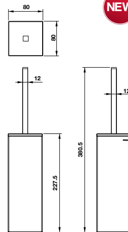
Giá treo cọ vệ sinh mặt kính trắng Toilet brush holder white glass
