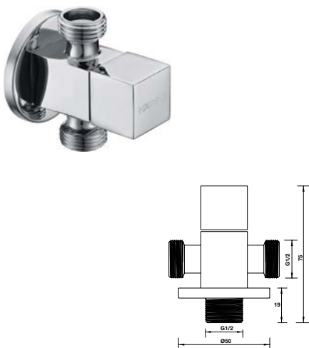
Van khóa nước dạng vuông 2 đường nước Square stop valve 2 outlets
