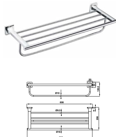
Kệ để khăn tắm Towel rack
