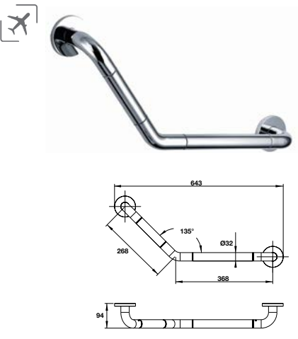
Tay vịn phòng tắm 110° 368 mm Handicapped 110° grab bar 368 mm
