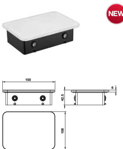
Kệ kính trắng 150 White glass shelf 150
