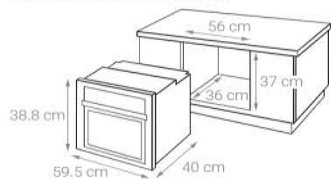
Kích thước lắp đặt lò vi sóng âm
