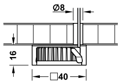
Surface mounting, square Lắp nổi, vuông
