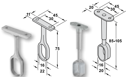
Rail centre support Giả đỡ thanh treo giữa
