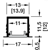
Routing dimensions Kích thước
