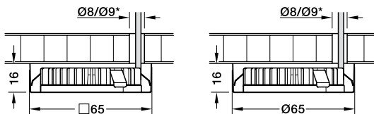
Surface mounting, square Lắp nổi, vuông
