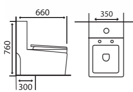
GMBC908 KT: 660 x 350 x 760 mm Giá: 6.170.000 Strap: 300 mm
