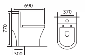
GMBC907 KT: 690 x 370 x 770 mm Giá: 4.900.000 Strap: 300 mm
