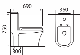
GMBC903 KT: 690 x 360 x 750 mm Giá: 4.500.000 Strap: 300 mm
