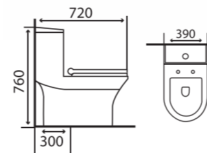
GMBC931 KT: 720 x 390 x 760 mm Giá: 5.000.000 Strap: 300 mm
