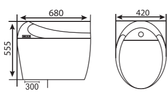
GMBC605 KT: 680 x 420 x 555 mm Giá: 26.200.000 Strap: 300 mm Không cắm biến
