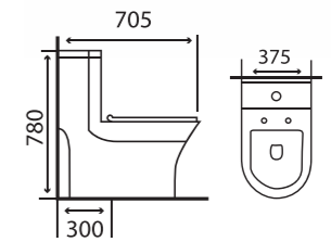
GMBC930 KT: 705 x 375 x 780 mm Giá: 5.170.000 Strap: 300 mm
