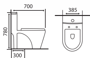
GMBC900 KT: 700 x 385 x 780 mm Giá: 4.500.000 Strap: 300 mm
