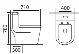
GMBC909 KT: 710 x 400 x 780 mm Giá: 5.170.000 Strap: 300 mm
