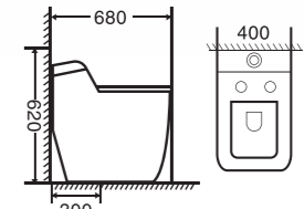
GMBC965 KT: 680 x 400 x 620 mm Giá: 8.000.000 Strap: 300 mm
