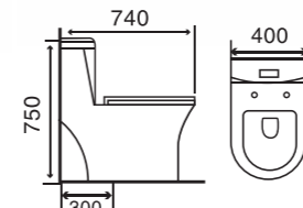
GMBC991 KT: 740 x 400 x 750 mm Giá: 4.900.000 Strap: 300 mm
