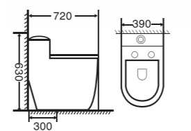
GMBC968 KT: 720 x 390 x 630 mm Giá: 5.500.000 Strap: 300 mm
