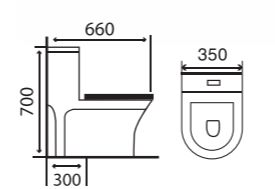
GMBC993 KT: 660 x 350 x 700 mm Giá: 4.400.000 Strap: 300 mm
