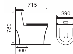
GMBC961 KT: 715 x 390 x 780 mm Giá: 4.800.000 Strap: 300 mm
