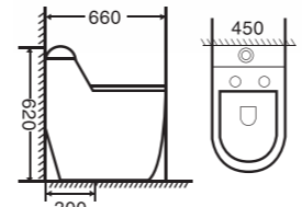
GMBC966 KT: 660 x 450 x 620 mm Giá: 8.000.000 Strap: 300 mm
