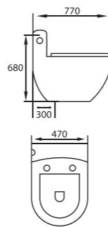
GMBC938 KT: 770 x 470 x 680 mm Giá: 8.800.000 Strap: 300 mm
