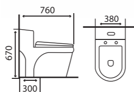
GMBC906 KT: 760 x 380 x 670 mm Giá: 5.050.000 Strap: 300 mm
