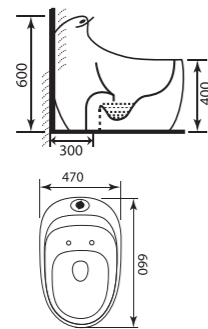
GMBC936 KT: 660 x 470 x 600 mm Giá: 7.500.000 Strap: 300 mm
