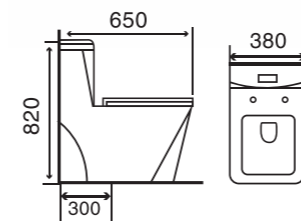
GMBC999 KT: 650 x 380 x 820 mm Giá: 5.200.000 Strap: 300 mm
