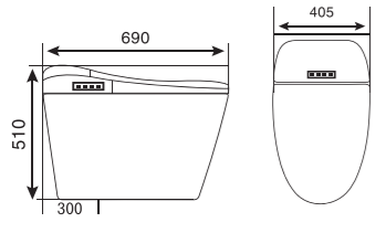
GMBC913 KT: 690 x 405 x 510 mm Giá: 38.000.000 Strap: 300 mm Cắm biến chân
