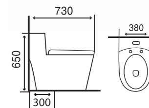
GMBC937 KT: 730 x 380 x 650 mm Giá: 6.170.000 Strap: 300 mm
