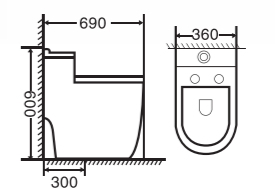
GMBC967 KT: 690 x 360 x 600 mm Giá: 5.100.000 Strap: 300 mm
