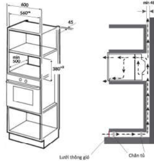
Lưới thông gió Chân tủ
