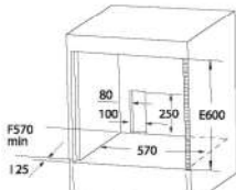
Kích thước khoét gỗ
